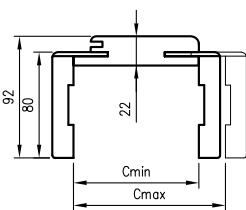
Przekrój OR z ką. T80
